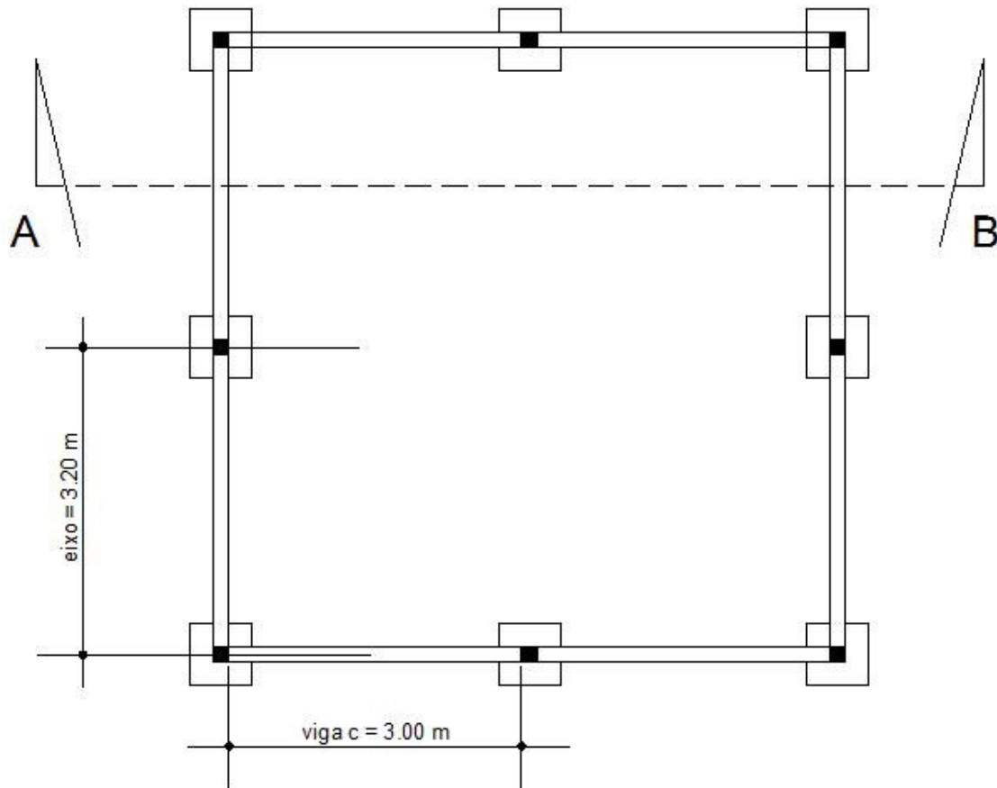
PLANTA
